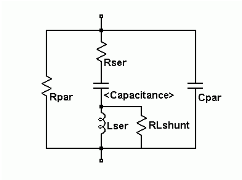
Capacitor Instance Parameters
